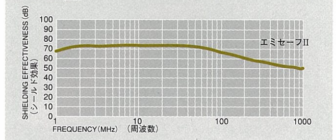
EMIシールド性能
