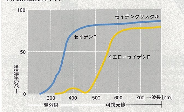
全分光線透過率グラフ
