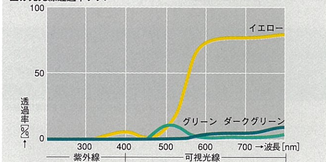
全分光線透過率グラフ
