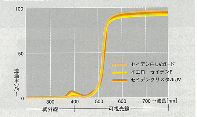
全分光光線透過率グラフ
